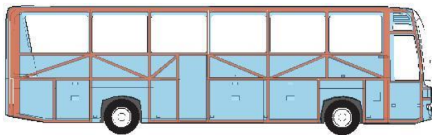
Рисунок 6.3 – Конструкції кузова туристичних автобусів, одно-і двоповерхові
