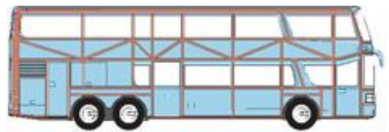
Рисунок 6.3 – Конструкції кузова туристичних автобусів, одно-і двоповерхові
