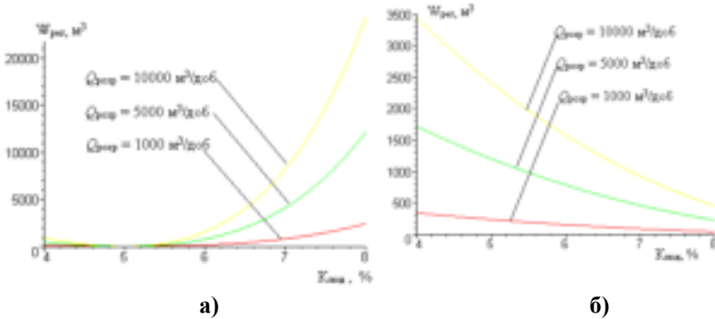
Рисунок 1 – Залежність регулюючого об'єму ПВ W_{\text{рег}} від коефіцієнту максимальної годинної подачі води до ПВ K_{\text{под}} (4 – 8 %) для значень розрахункових витрат Q_{\text{розра}} = 1000 \text{ м}^3/\text{доб} , 5000 \text{ м}^3/\text{доб} та 10000 \text{ м}^3/\text{доб} при значенні коефіцієнта максимального годинного забору води з ПВ: а) K_{\text{заб}} = 5 \% ; б) K_{\text{заб}} = 10,4 \%
