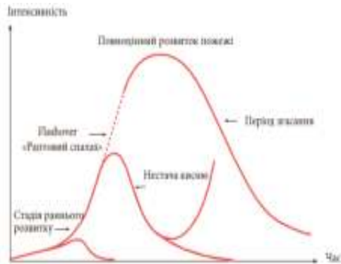
Рисунок 1 – Крива розвитку пожежі в огороженні
