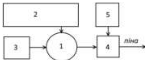
Рисунок 1 – Схема отримання газонаповненої піни: 1 – насос; 2 – цистерна для води; 3 – змішувач з піноутворювачем; 4 – пінозмішувач; 5 – компресор (балони зі стисненим повітрям)
