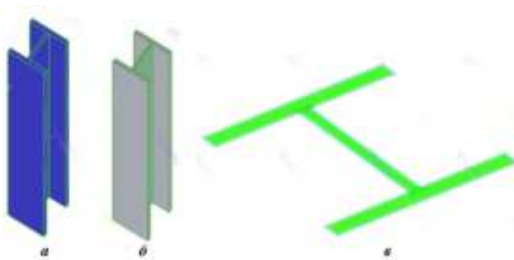
Рисунок 1 – Кінцево-елементна модель вогнезахисної сталевій колони в 3D (а, б) та 1D (в) постановці
