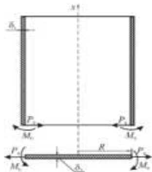
Рисунок 1 – Крайові сили в стінці циліндричного резервуара та на круглому дні
