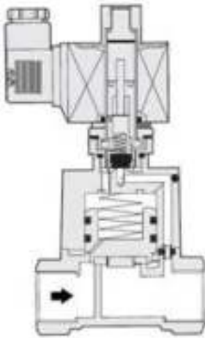
Рисунок 1 – Будова електромагнітного клапана постійно відкритого типу
