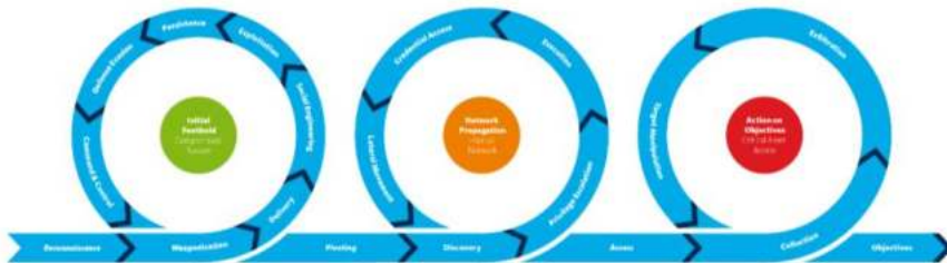
Рисунок 2 – Етапи ланцюга Unified Kill Chain
