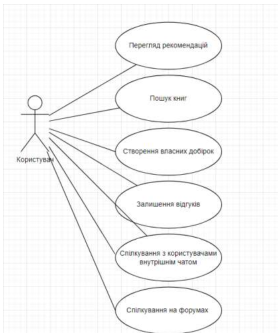
Рисунок 2 – Діаграма прецедентів
