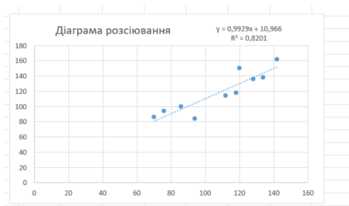
Рисунок 2 – Діаграма розсіювання
