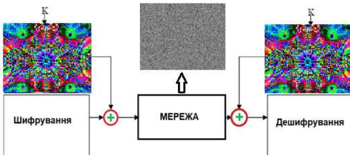
Рисунок 1 – Процес фрактального шифрування (К-ключ)
