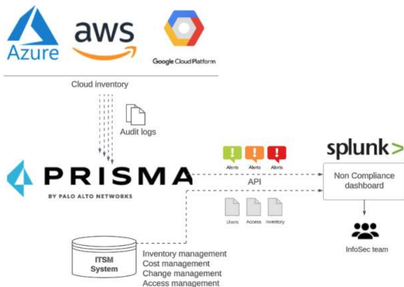
Рисунок 1 – Схема процесу сканування конфігурацій
