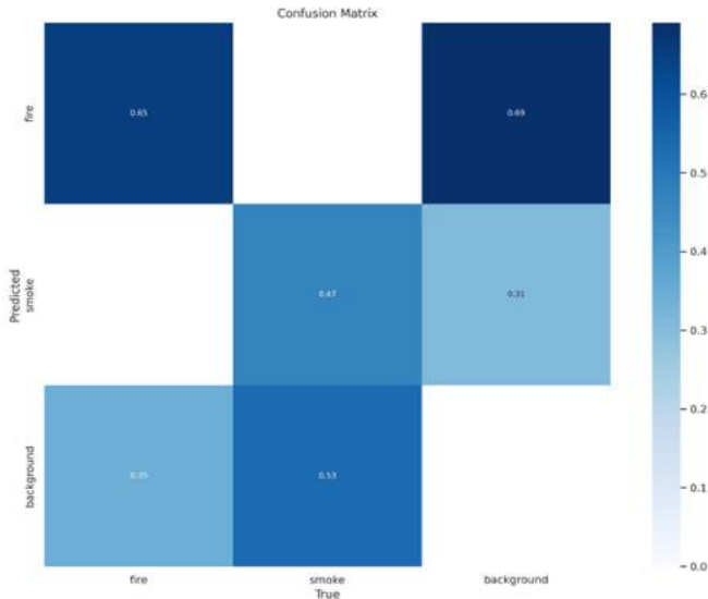
Рисунок 3 – Матриця плутанини
