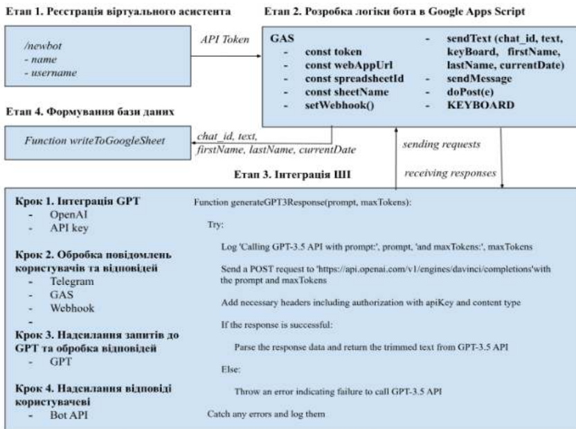
Рисунок 1 – Схема реалізації методу удосконалення роботи СМО з використанням ВА на базі III
