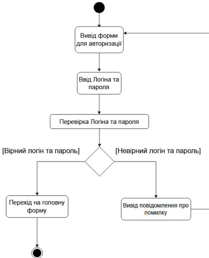
Рисунок 2 – Діаграма діяльності для форми авторизації користувачів інформаційної системи
