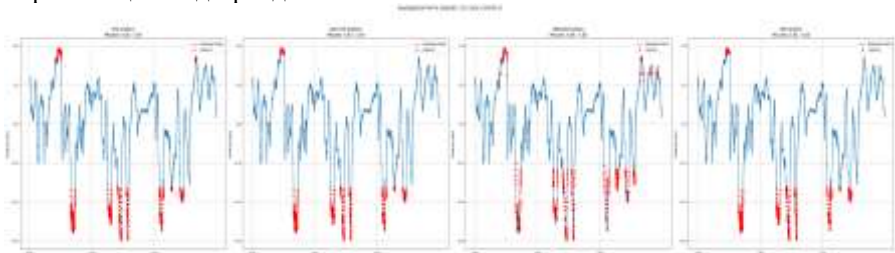
Рис. 3. Результати пошуку викидів за допомогою методів STD, STD з логарифмічною трансформацією, DBSCAN та IQR
