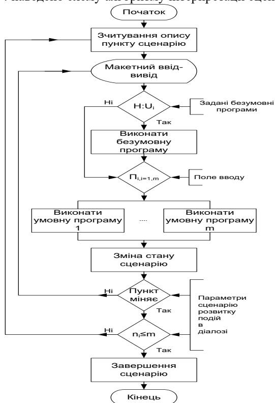
Рис. 4. Алгоритм інтерпретації табличного сценарію
