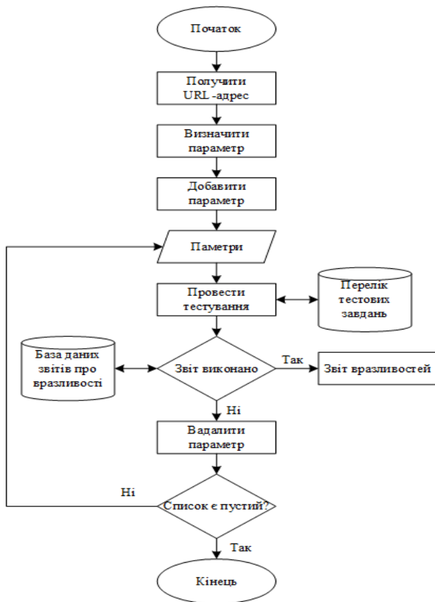
Рис. 1. Алгоритм автоматизованого пошуку SQL-ін'єкцій у проєктованій системі
