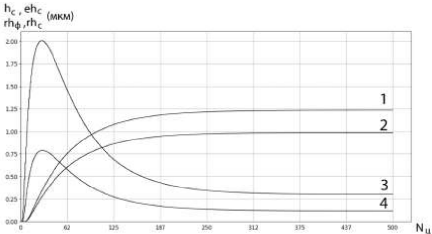
Рисунок 2 – Перехідні процеси товщин фарби і зволожувального розчину (1 – емульгована фарба, 2 – фарба без зволоження; розчин: 3 – на формі, 4 – відбитках).
