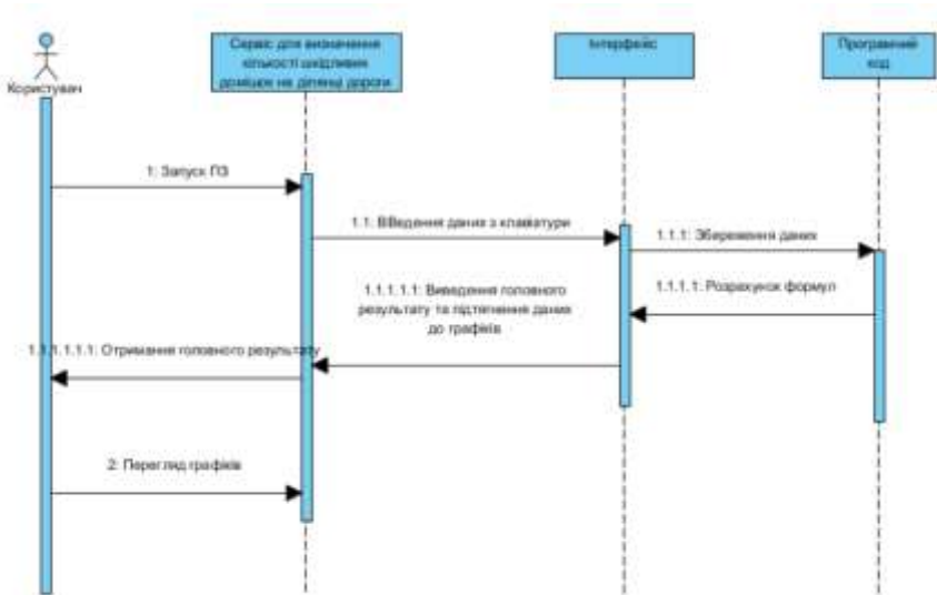
Рис.2 Діаграма послідовності для введення даних у програмному забезпеченні
