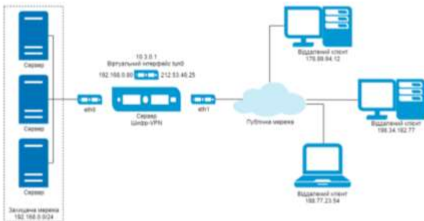
Рисунок 3 – Структурна схема мережі VPN організацій
