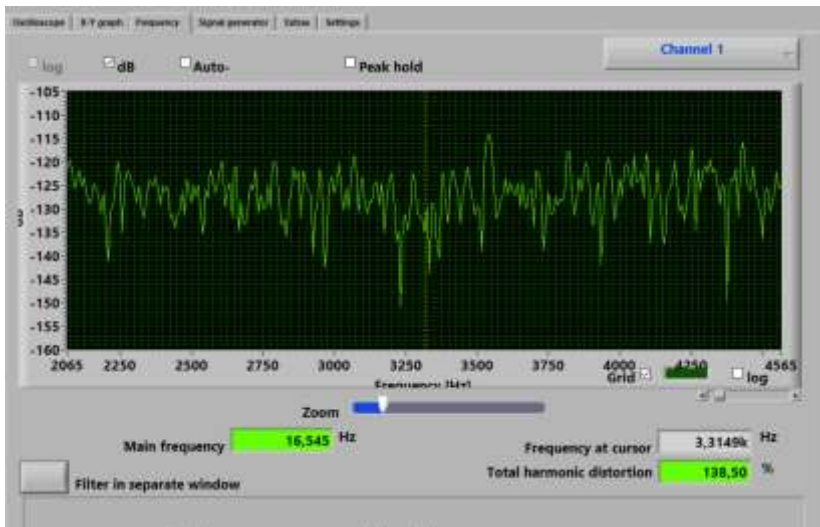
Рис.3. Скріншот акустичних сигналів в режимі реального часу на осцилографі
