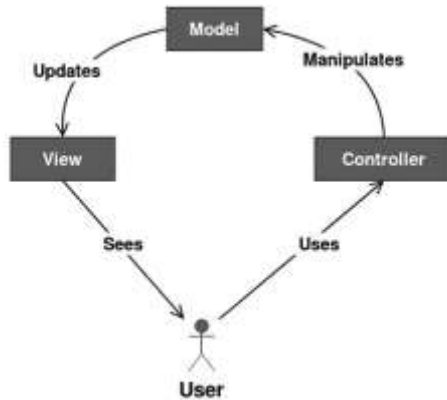
Рис. 1 – Графічне представлення типової структури MVC архітектури
