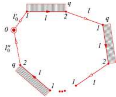
Рисунок 2 – Схема-розгортка маятничого циклу
