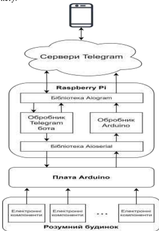
Рис. 1. Загальна схема системи обміну повідомленнями
