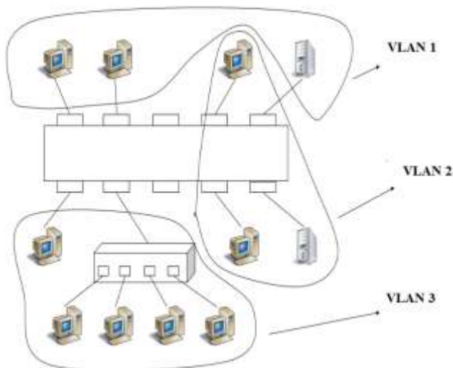
Рисунок 1 – Побудова VLAN на базі одного комутатора способом групування портів
