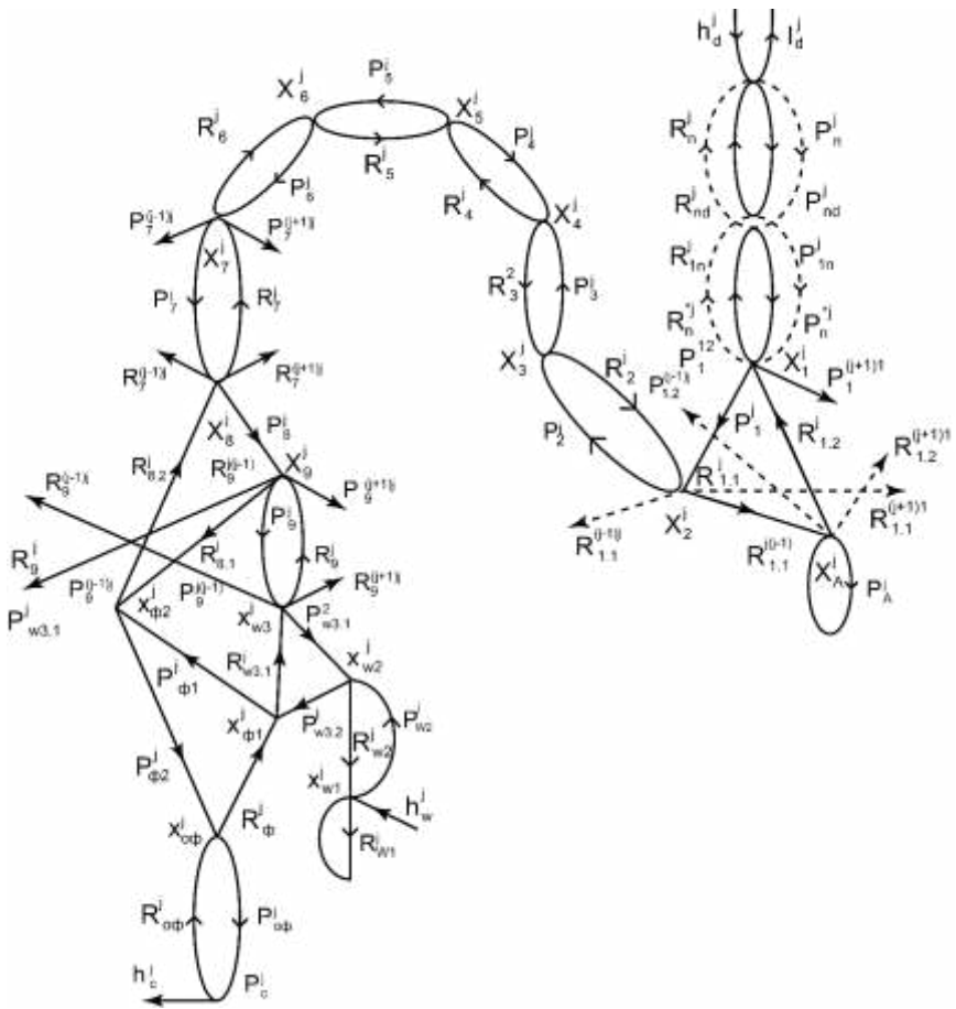
Рисунок 1 – Сигнальний граф j -тої зони фарбодрукарської системи
