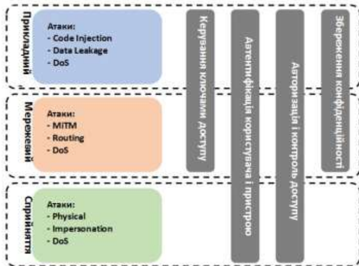
Рисунок 1. Рівні IoT з категоріями атак та їх контрзаходами [1]
