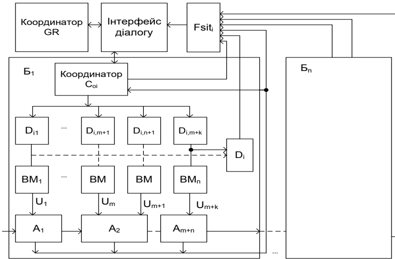
Рис. 4. Схема ділового управління з координатором в ієрархічній системі.
