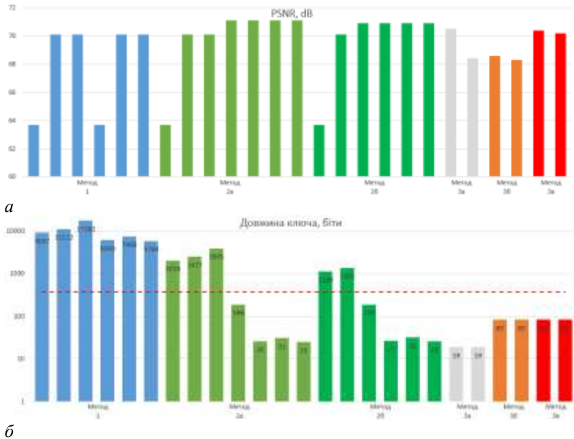
Рис. 3. Порівняння ефективності різних стеганографічних методів для S_p «sat.jpg» (алгоритм Кенні, c_T = 0,15, k_T = 0,5 , різні значення L_T ) у випадку 368-бітного повідомлення M_T : a – похибки вбудованого контейнера S_p за піковим співвідношенням сигналу до шуму; б – реальні довжини стеганоключа K_T
