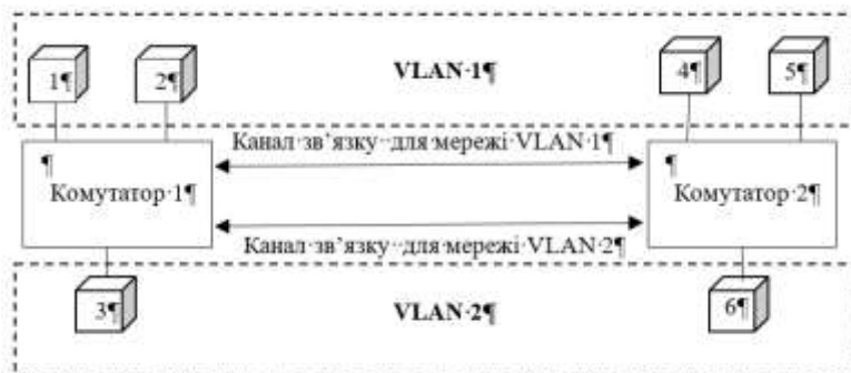
Рисунок 2 – Мережі VLAN на базі декількох комутаторів без магістрального з'єднання
