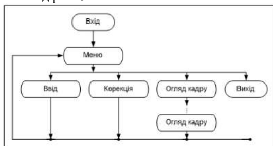
Рис. 3. Структура сценарію діалогу
