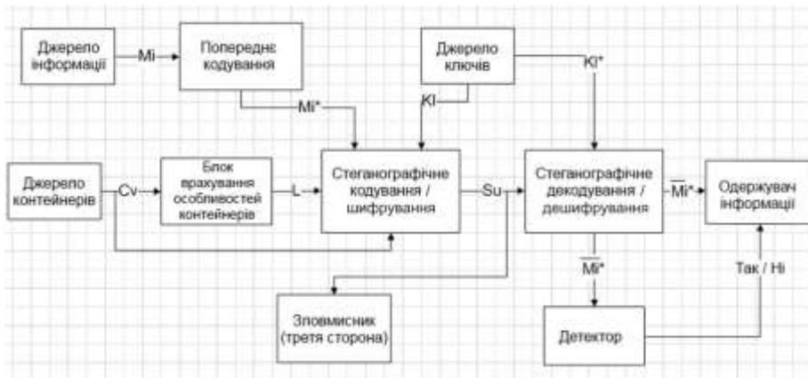
Рис. 1. Базова математична модель стеганосистеми
