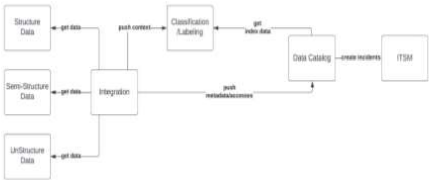
Рис. 1. Потік даних при обробці та класифікації інформації
