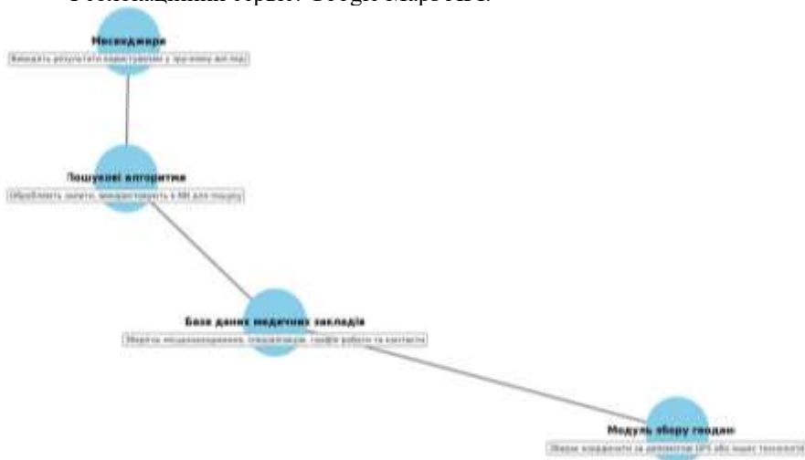
Рис. 1. Архітектура сервісу.
