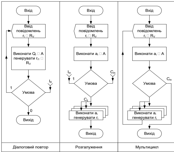
Рис. 2. Схеми діалогових управляючих конструкцій
