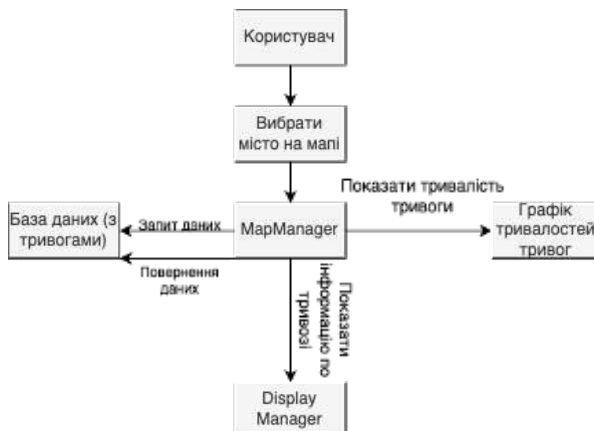
Рисунок 2 – Діаграма послідовностей для Мапи тривог
