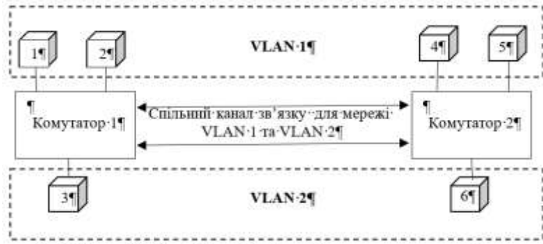
Рисунок 3 – Мережі VLAN на базі декількох комутаторів з магістральним з’єднанням
