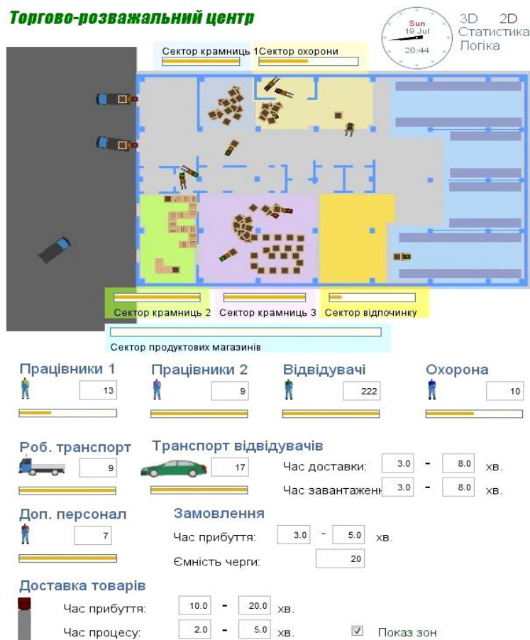
Рис. 4.4.1. Імітаційна модель життєвого циклу проекту створення об'єкта з масовим перебуванням людей
