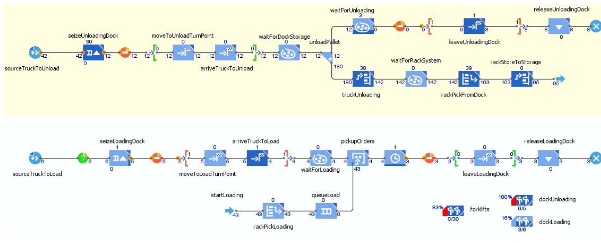
Рис. 4.4.2. Динамічна модель імітаційного середовища життєвого циклу об'єктів з масовим перебуванням людей
